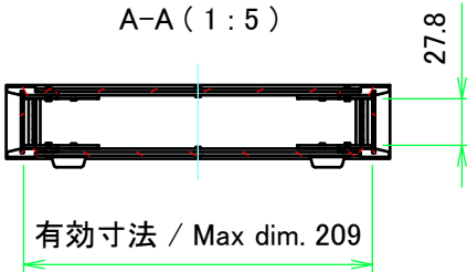
A-A ( 1 : 5 )
