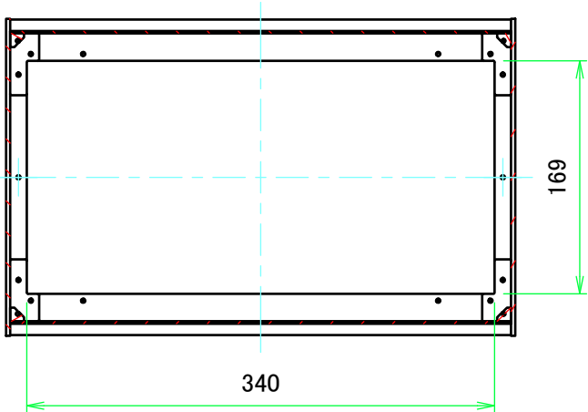
B-B ( 1 : 5 )
