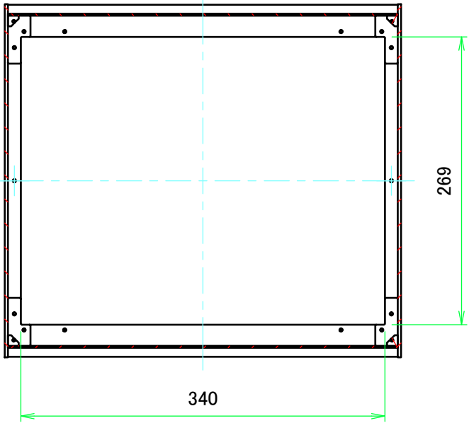
B-B ( 1 : 5 )
