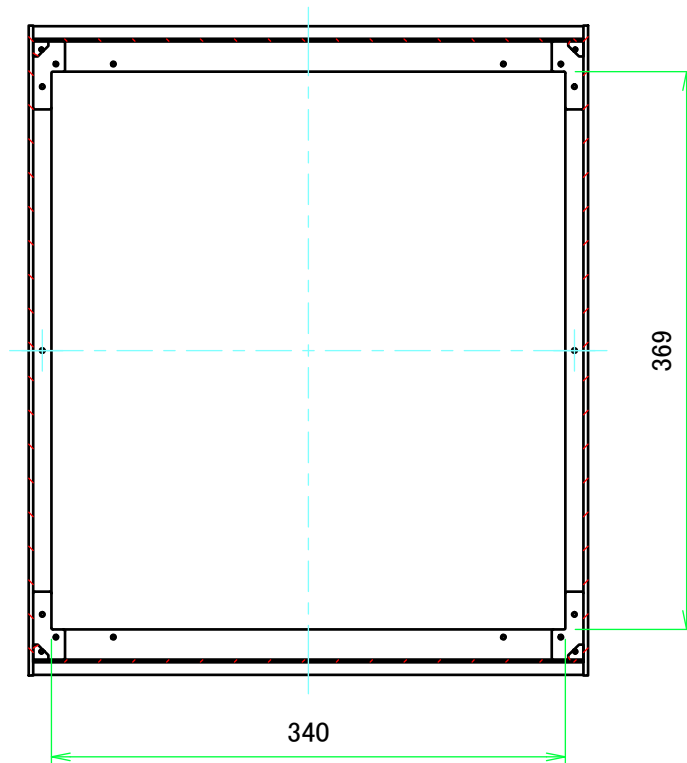
B-B ( 1 : 5 )
