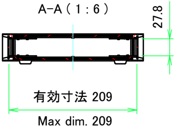
A-A ( 1 : 6 )
