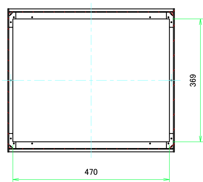
B-B ( 1 : 7 )
