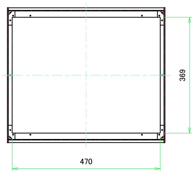
B-B ( 1 : 7 )
