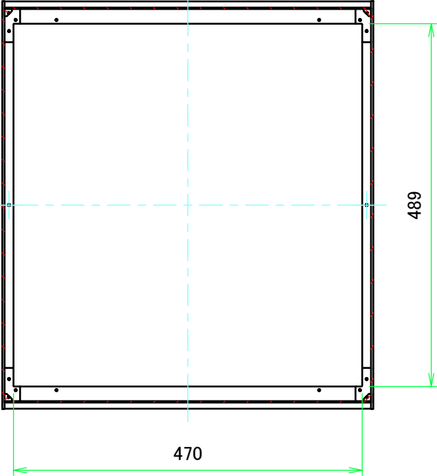
B-B ( 1 : 7 )
