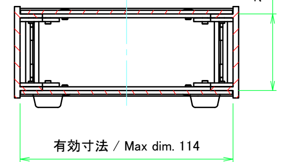
C-C ( 1 : 2 )
