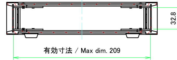
A-A ( 1 : 3 )
