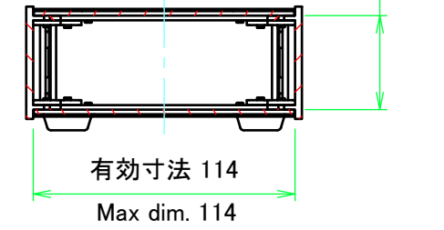
C-C ( 1 : 3 )
