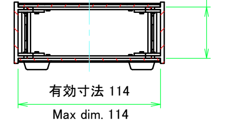
C-C ( 1 : 3 )
