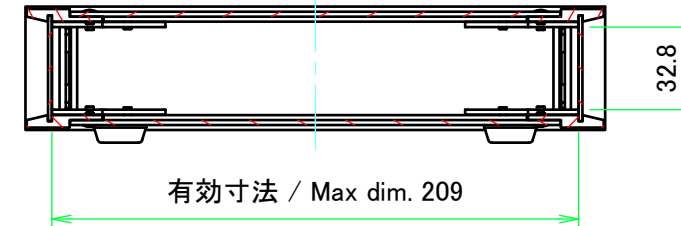
A-A ( 1 : 3 )
