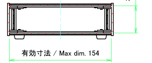
C-C ( 1 : 3 )
