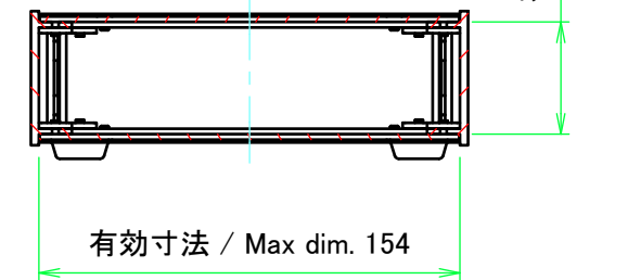
C-C ( 1 : 3 )
