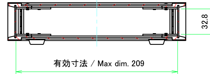
A-A ( 1 : 3 )
