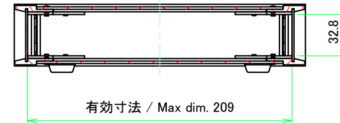
A-A (1:3)
