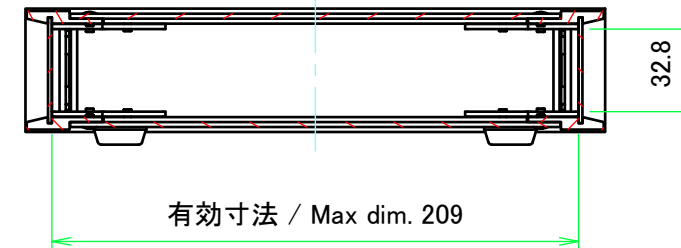
A-A (1:3)
