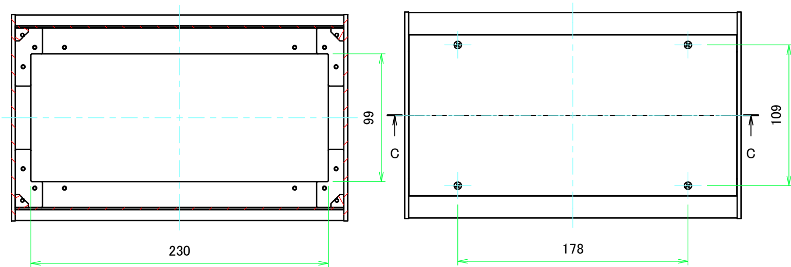
B-B ( 1 : 3 )
