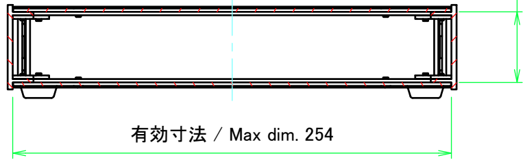
C-C ( 1 : 3 )
