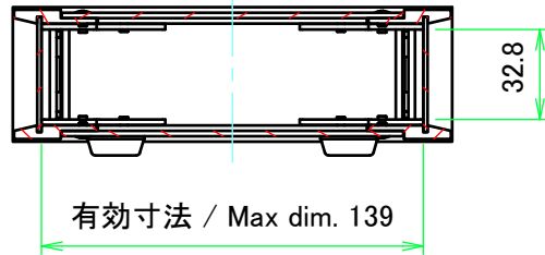
A-A ( 1 : 3 )
