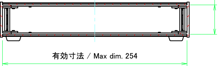
C-C ( 1 : 3 )
