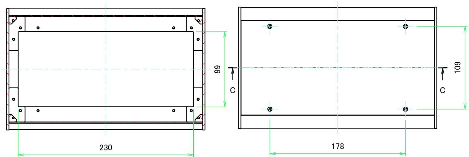
B-B ( 1 : 3 )
