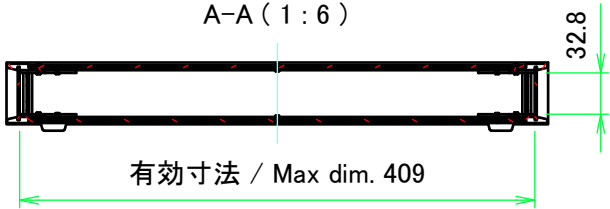
A-A ( 1 : 6 )
