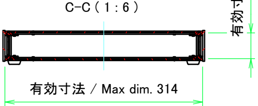
C-C ( 1 : 6 )
