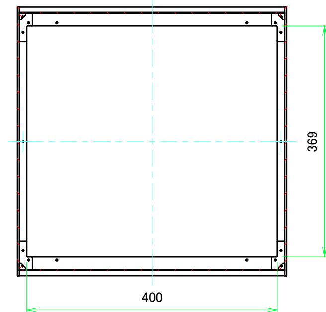
B-B ( 1 : 6 )
