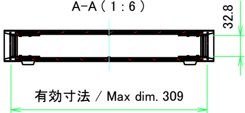
A-A (1:6)
