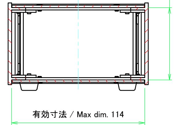
C-C (1:2)
