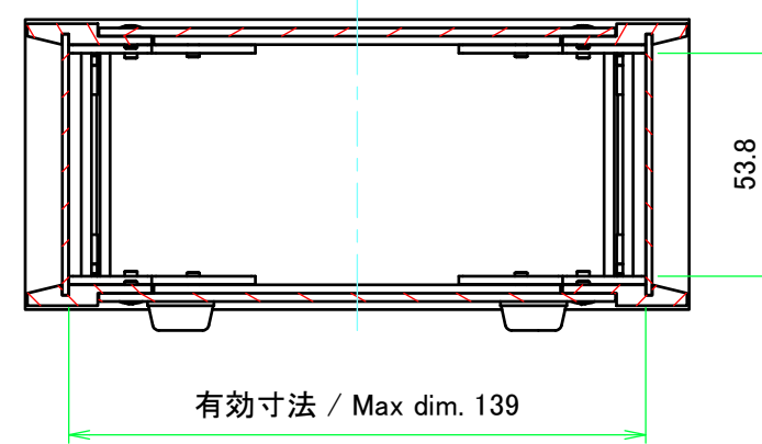
A-A (1:2)
