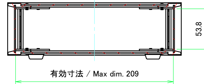
A-A ( 1 : 3 )
