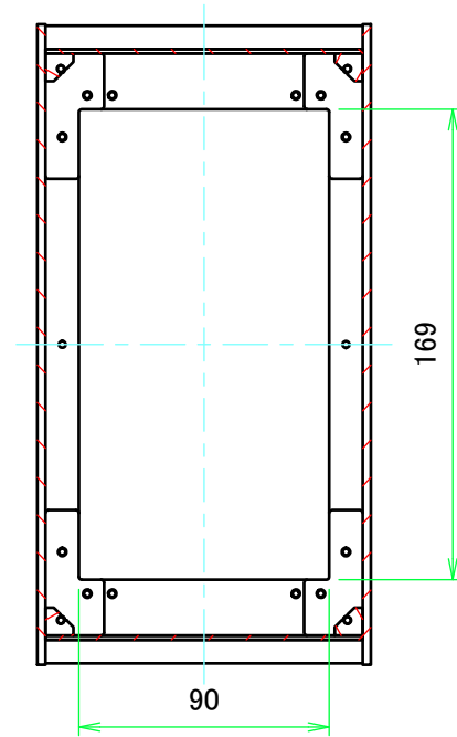
B-B ( 1 : 3 )
