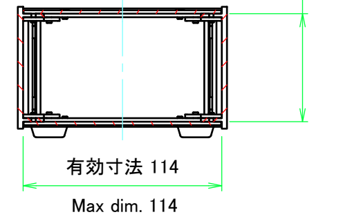
C-C ( 1 : 3 )
