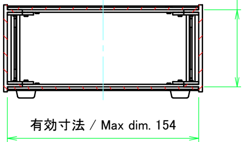
C-C ( 1 : 3 )
