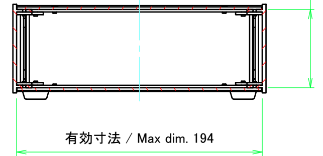
C-C ( 1 : 3 )
