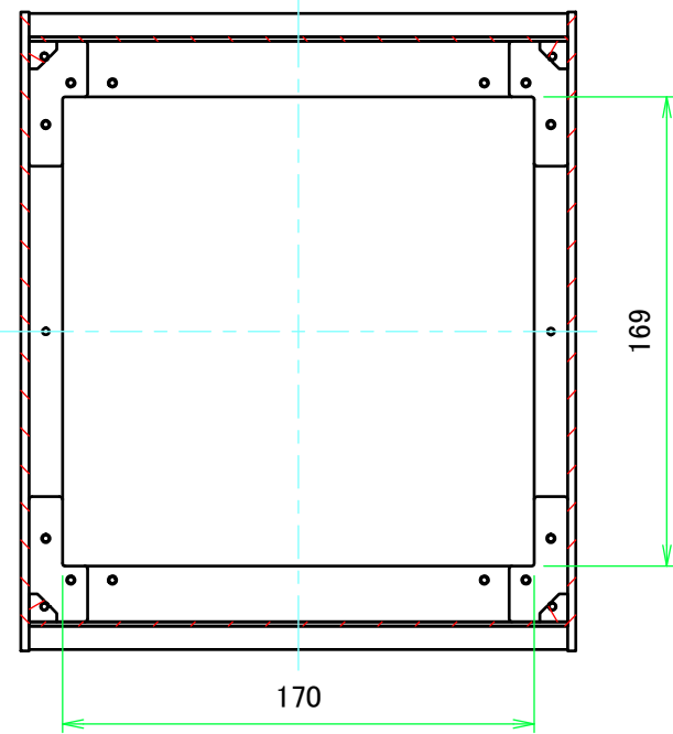
B-B ( 1 : 3 )
