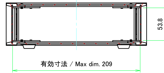
A-A ( 1 : 3 )
