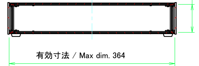
C-C ( 1 : 5 )
