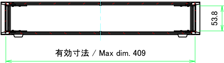
A-A ( 1 : 5 )
