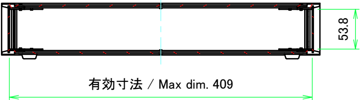
A-A ( 1 : 5 )
