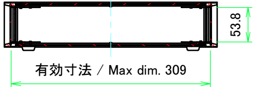
A-A ( 1 : 6 )
