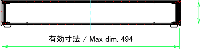
C-C ( 1 : 6 )
