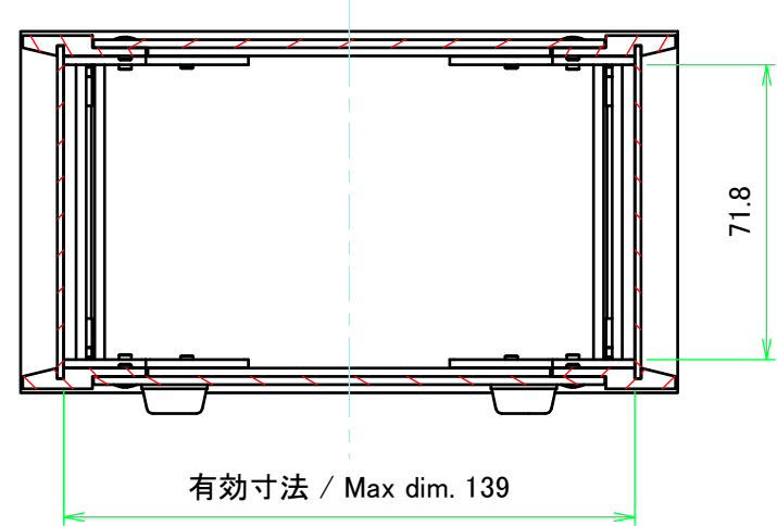
A-A ( 1 : 2 )
