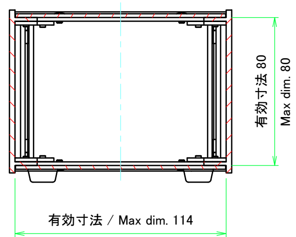
C-C ( 1 : 2 )
