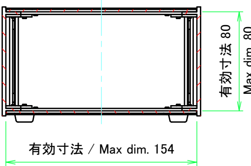
C-C ( 1 : 3 )
