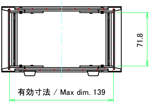
A-A ( 1 : 3 )
