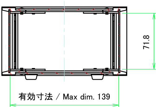
A-A (1:3)
