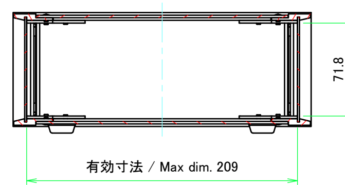
A-A (1:3)
