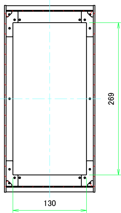
B-B ( 1 : 4 )
