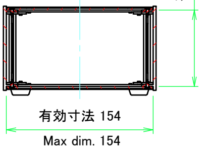
C-C ( 1 : 4 )
