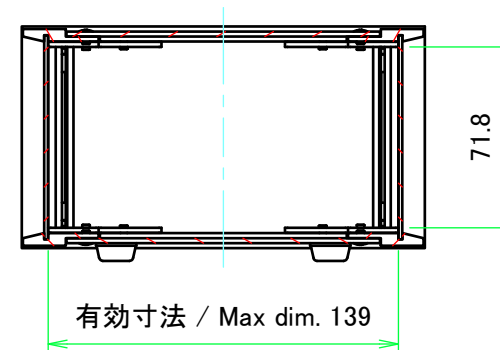
A-A (1:3)
