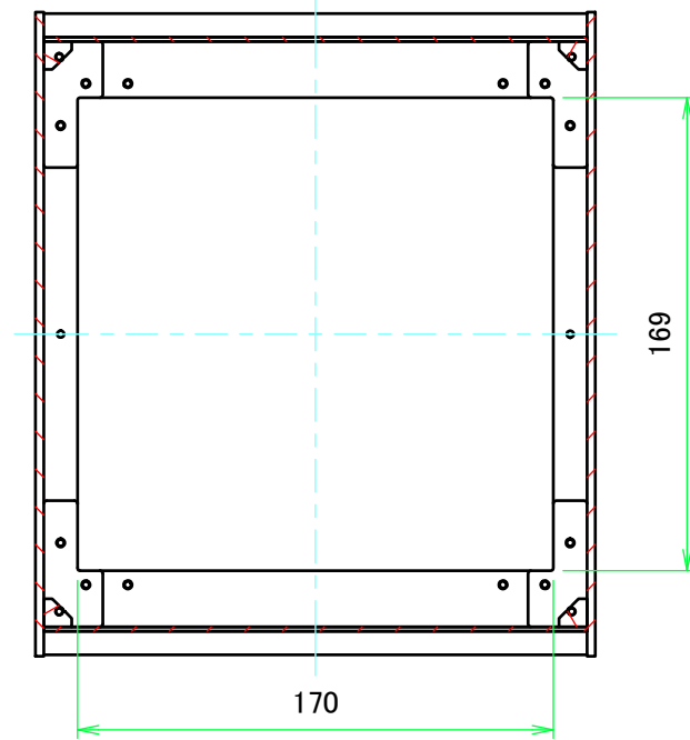
B-B ( 1 : 3 )
