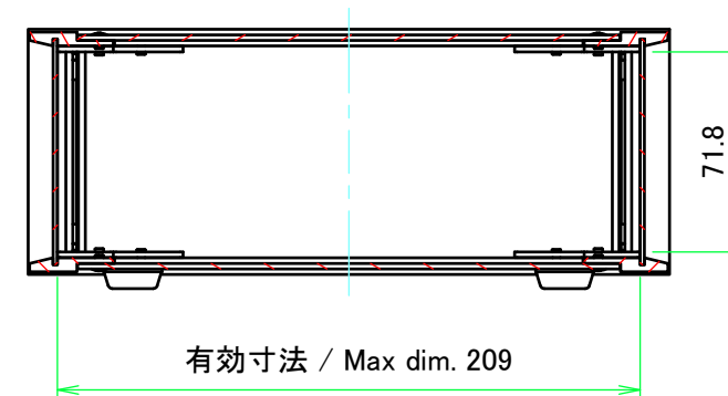
A-A ( 1 : 3 )
