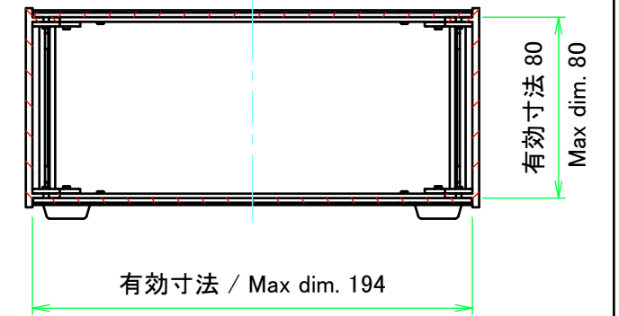
C-C ( 1 : 3 )
