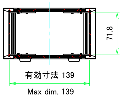
A-A ( 1 : 4 )
