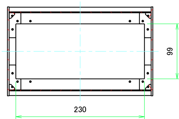
B-B ( 1 : 4 )
