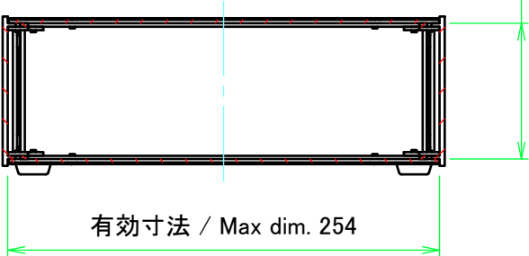
C-C ( 1 : 4 )
