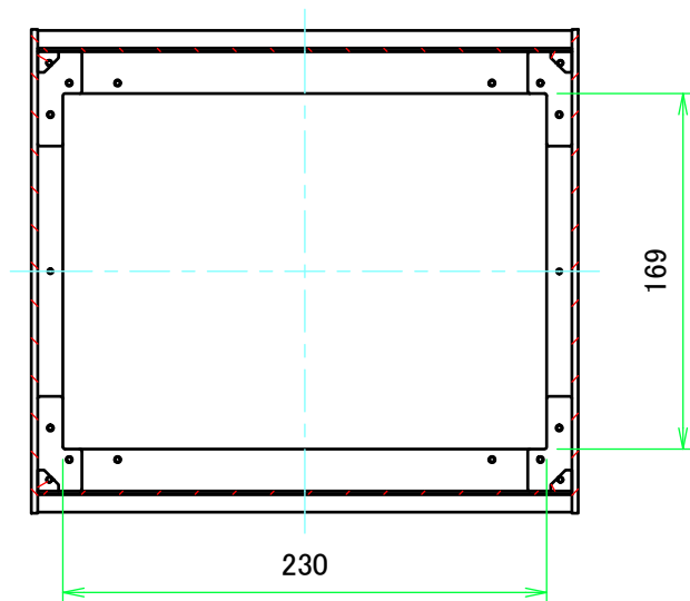
B-B ( 1 : 4 )
