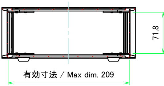
A-A ( 1 : 4 )
