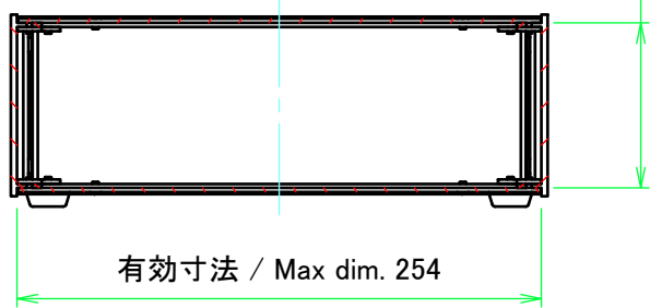
C-C ( 1 : 4 )
