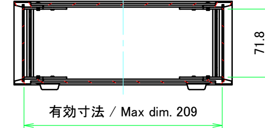
A-A ( 1 : 4 )
