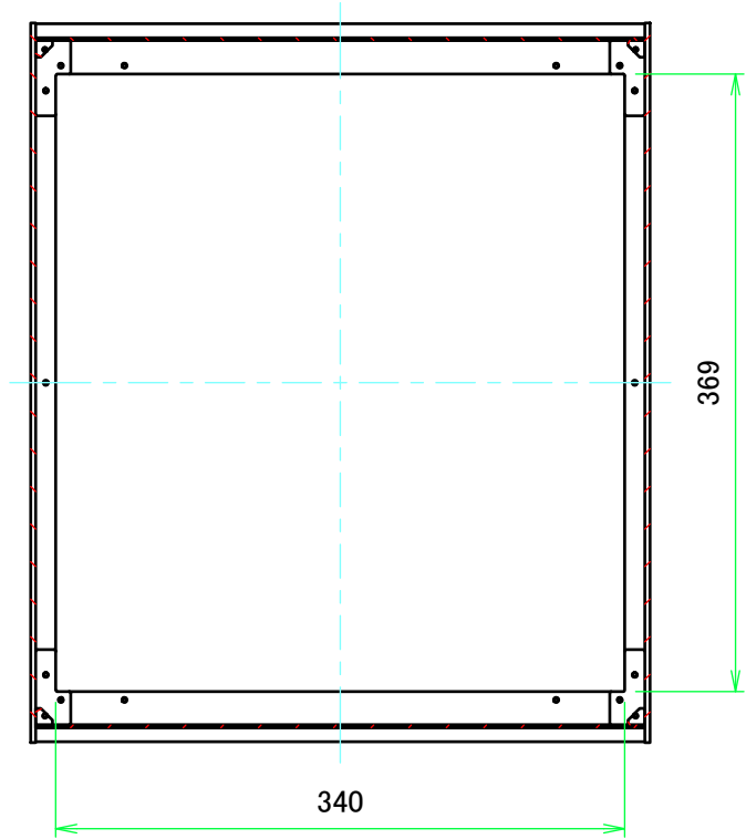
B-B ( 1 : 5 )
