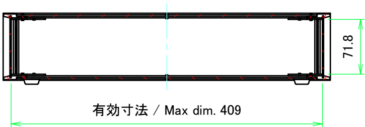
A-A ( 1 : 5 )
