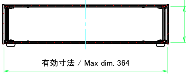
C-C ( 1 : 5 )
