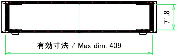
A-A ( 1 : 6 )
