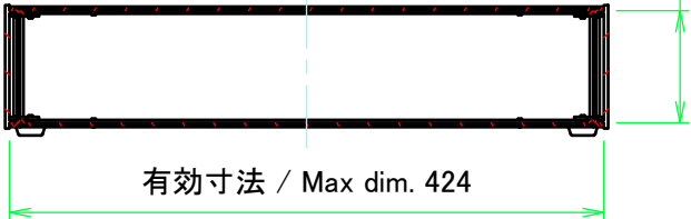
C-C ( 1 : 6 )
