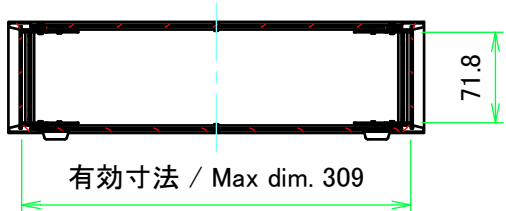
A-A ( 1 : 6 )
