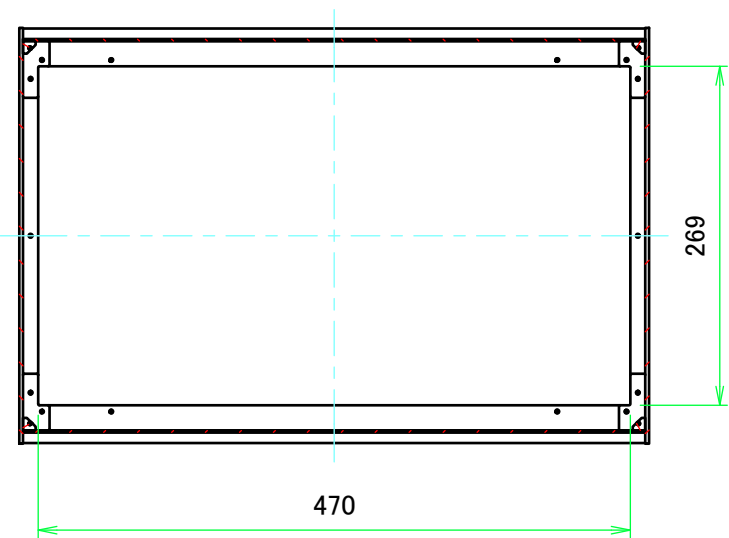
B-B ( 1 : 6 )
