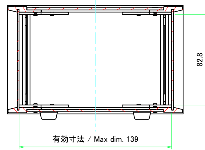
A-A (1:2)
