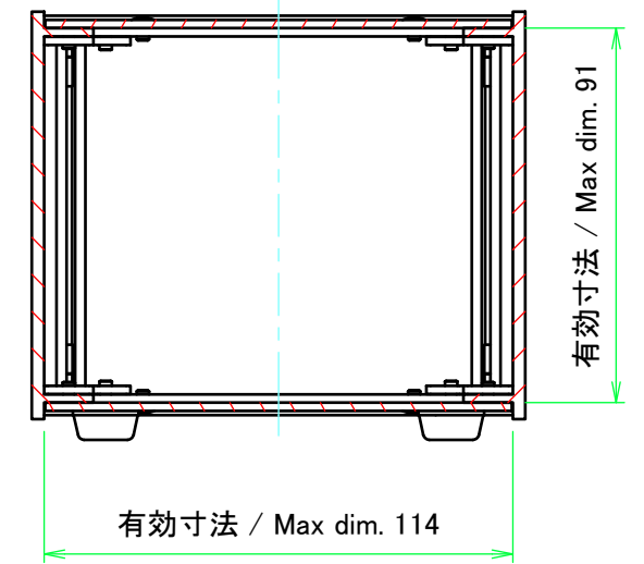
C-C (1:2)
