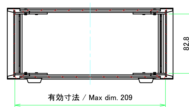
A-A ( 1 : 3 )
