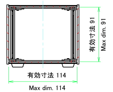
C-C ( 1 : 3 )
