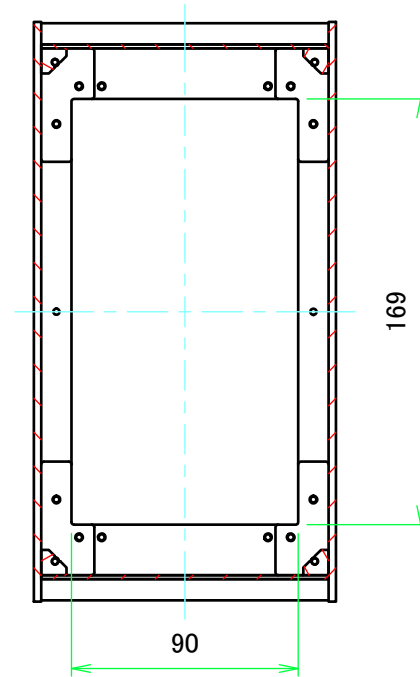
B-B ( 1 : 3 )
