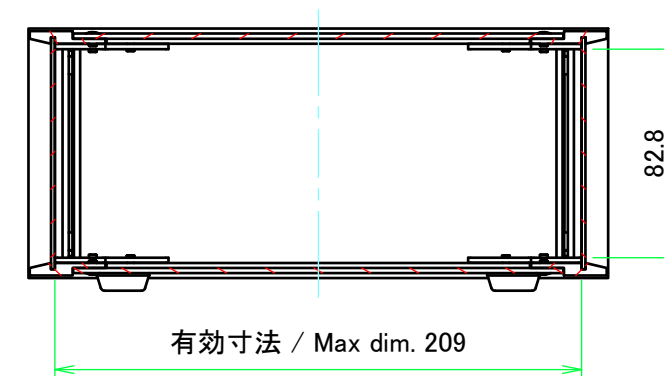
A-A ( 1 : 3 )
