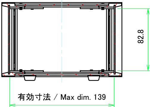
A-A (1:3)
