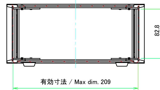
A-A (1:3)
